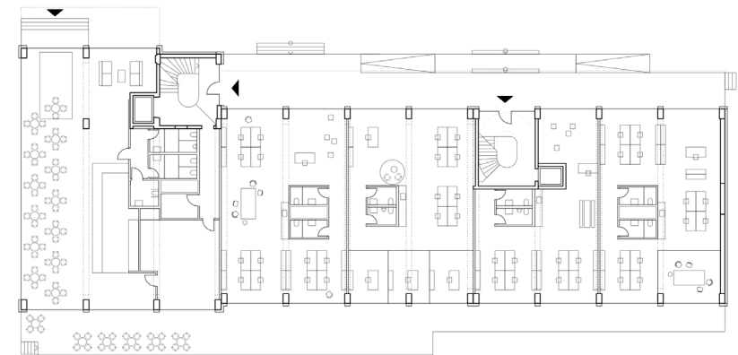
Grundrisse EG und 1. OG
