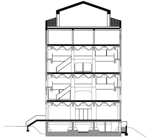
Schnitt nördlicher Teil (BT2, neuerer Teil), M1:500
