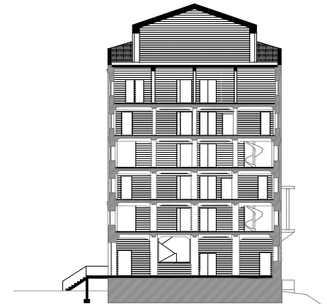
Schnitt Mitte (BT1 älterer Teil) M1:500
