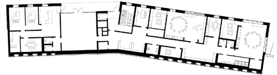
Grundriss EG
