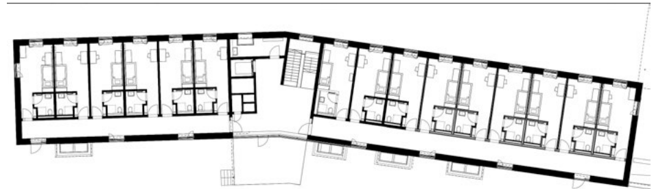
Grundriss OG
